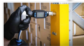
Digitale Drehmoment- Adapter | 12,5 mm (1/2") | 40 - 200 Nm
